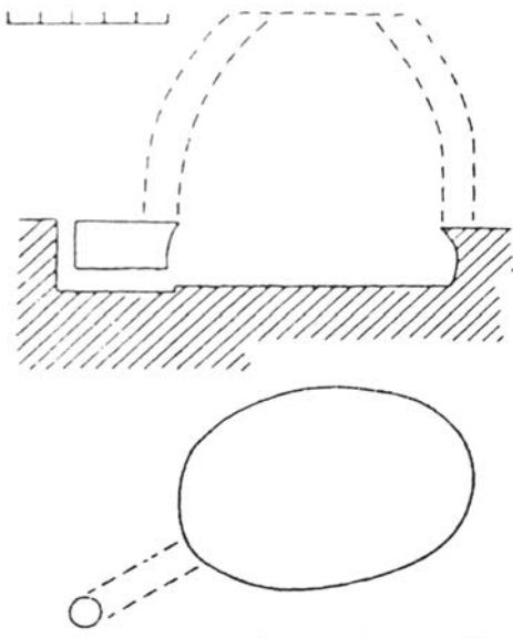
İlk Tunc dövrü metaləritmə sobası. Babadərviş (Махмудов Ф.Р., Мунчаев Р.М., Нариманов, 1968).
