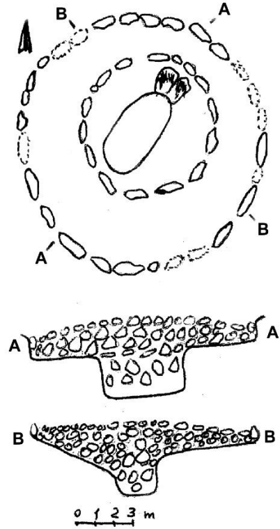
Şəkil 3. 4 saylı kromlextli Nəhəcir kurqanının planı
