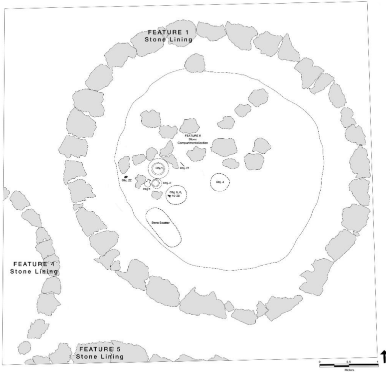
Şəkil 1. Qızqala kurqanlarından birinin planı.
